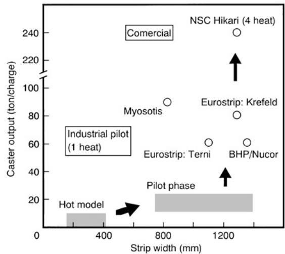
図7 ストリップ連続 casting プラントの開発状況
