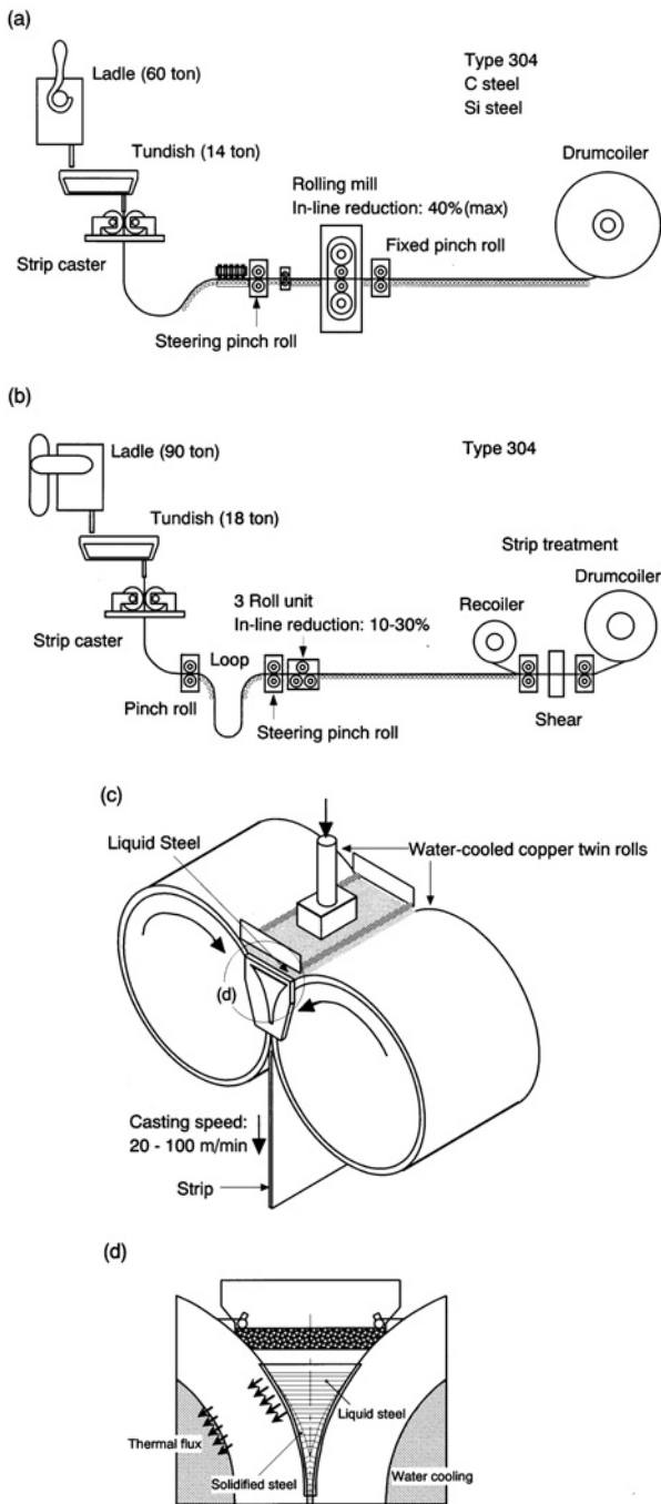
図5 ストリップ連続 casting ラインの概念図 (a) Terni PP, (b) Krefeld PIP, (c) 双ロール法概念図, (d) 铸造部拡大図
