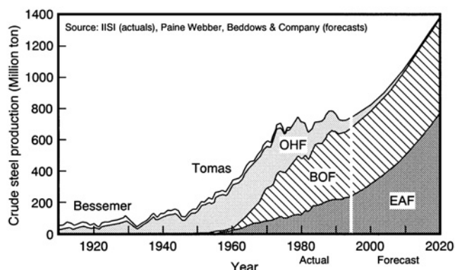
図12 世界の粗鋼生産量予測(製鋼法別) EAF: 電気炉, BOF: LD 転炉, OHF: 平炉
